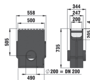
studzienka z ocynkowanym osadnikiem, z rusztem kratowym MW 30/30, kl. B 125
