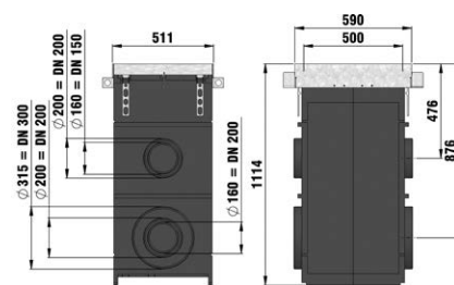
studzienka z rusztem żeliwnym, szczelinowym, kl. E 600
