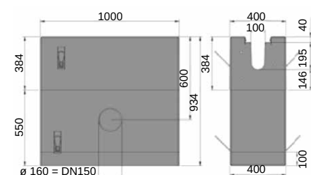
studzienka, 2-częściowa, z ocynk. osadnikiem i mufą połączeniową DN 150
