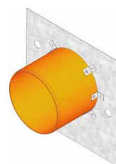
ścianka czołowa typ 010, z króćcem z tworzywa DN 100
