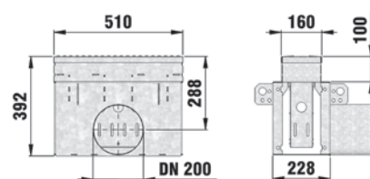
studzienka z ocynkowanym osadnikiem
