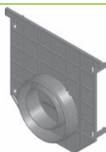
ścianka czołowa typ 01, z uformowa- nym króćcem DN 70/100, tworzywo
