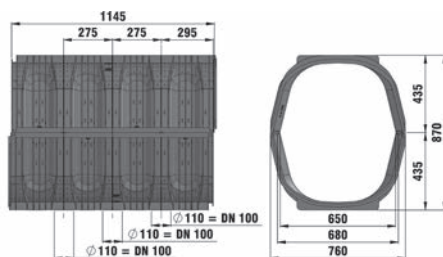
TWIN 1/1, czarny (2 część. 506 l), perforowany
