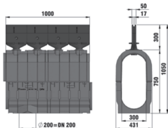
typ G 8300, szczelina 17 mm , KTL
