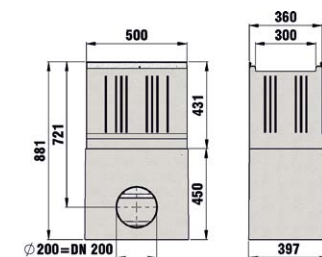
studzienka 2-cz. z ocynkowanym osadnikiem
