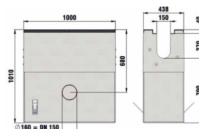
studzienka 2-częściowa, z ocynk. osadnikiem, z mufą połączeniową DN 150
