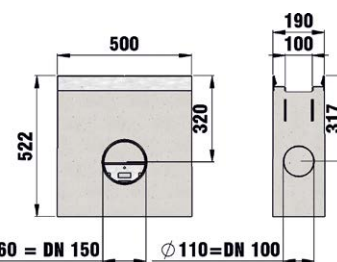
studzienka z ocynkowanym osadnikiem, ramy ze stali ocynk.
