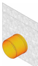
ścianka czołowa typ 01, z króćcem z tworzywa DN 200, ocynk.
