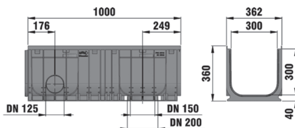
typ 010, z rusztem żeliwnym, szczelinowym G-TEC, z powłoką KTL
