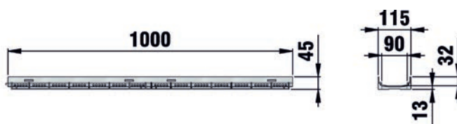
korytko typ 45, z tworzywa, w kolorze srebrnym
