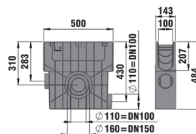
studzienka z osadnikiem z tworzywa
