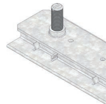
zestaw do regulacji wysokości DACHFIX STEEL 115, typ 45 (wymagane 2 szt. na m.b.)
