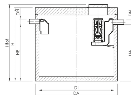
osadnik betonowy – przekrój
