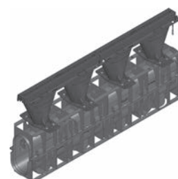
typ F 1200, szczelina 14 mm
