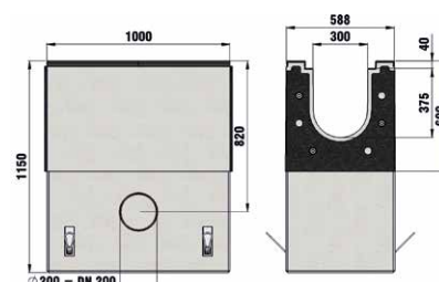
studzienka 2-częściowa, z ocynk. osadnikiem, z mufą połączeniową DN 200
