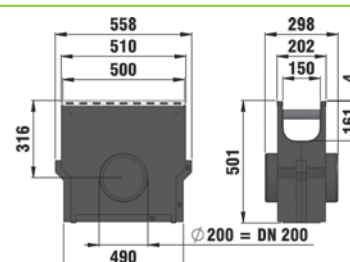
studzienka z ocynkowanym osadnikiem i ścianką czołową
