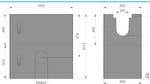
studzienka 2-częściowa, połączona fabrycznie z ocynk. osadnikiem, ramy ocynk., z mufą podłączeniową DN 200
