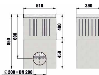
studzienka wielofunkcyjna, 2-częściowa, bez pokrywy
