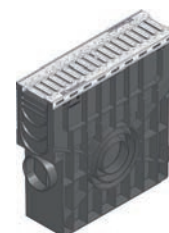
studzienka z osadnikiem z tworzywa, z rusztem szczelinowym SW 75/9, zaciskowym, przejezdny dla samochodów osobowych
