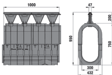
typ F 8200, szczelina 6 mm
