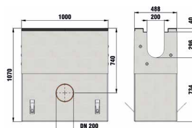
studzienka 2-częściowa, z ocynk. osadnikiem, z mufą połączeniową DN 200
