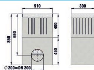
studzienka wielofunkcyjna 2-częściowa, z ocynkowanym osadnikiem, z rusztem żeliwnym, szczelinowym SW 2 x 140/20, czarnym, kl. F 900
