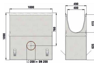
studzienka z ocynkowanym osadnikiem, typ 01
