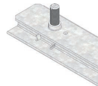
zestaw do regulacji wysokości DACHFIX STEEL 155, typ 45, ocynk. (wymagane 2 szt. na m.b.)
