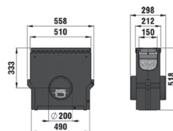
studzienka z ocynk. osadnikiem, z rusztem szczelinowym, poliamidowym FIBRETEC SW 9, kl. B 125
