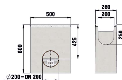
studzienka z ocynkowanym osadnikiem
