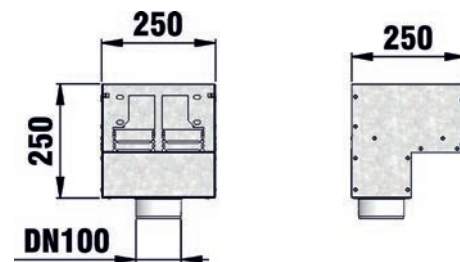
element odpływowy do typu 100, 150
