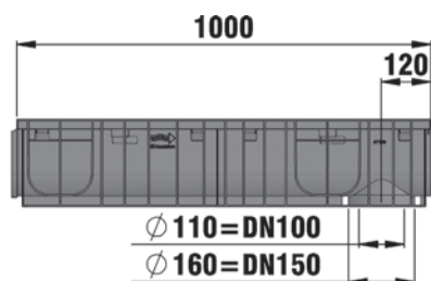
typ 01 z rusztem szczelinowym, poliamidowym FIBRETEC SW 9
