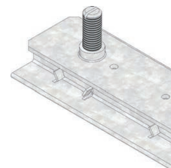
zestaw do regulacji wysokości DACHFIX STEEL 135, typ 45 (wymagane 2 szt. na m.b.)
