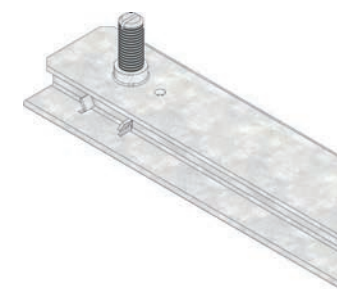
zestaw do regulacji wysokości DACHFIX STEEL 205, typ 45 (wymagane 2 szt. na m.b.)
