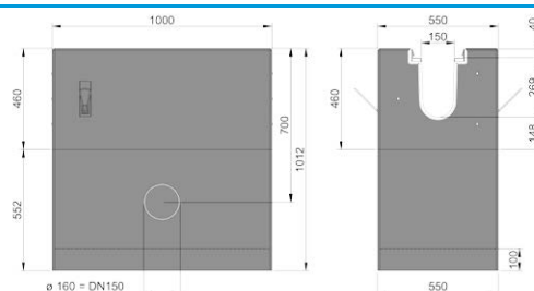
studzienka 2-częściowa, połączona fabrycznie z ocynk. osadnikiem, ramy ocynk., z mufą połączeniową DN 150
