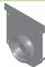
ścianka czołowa typ 01, z uformowanym króćcem DN 70/100, tworzywo
