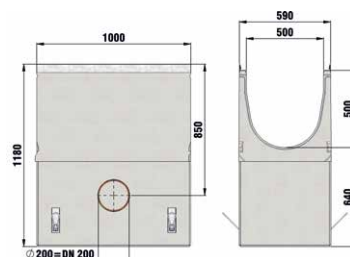
studzienka z ocynkowanym osadnikiem, typ 01
